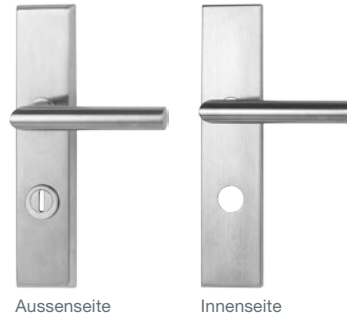
DRÜCKER- UND ZYLINDERGARNITUR Langschild Glutz 6150S.2 ES1, mit Zylinderschutz, Aussenseite Langschild Glutz 6146C.0 ES1, Innenseite Drücker Glutz 5071 Memphis Edelstahl matt
