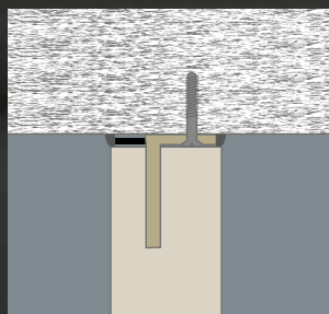
Verdeckte Montage
