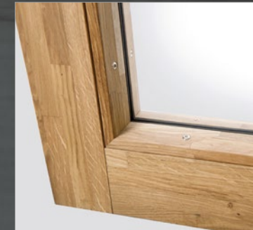
Beidseitig flächenbündige Glasleiste: geradlinige Optik für ein elegantes Erscheinungsbild
